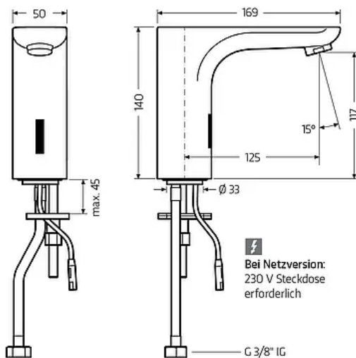
Armatur:
