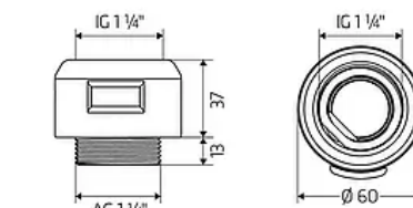
Elektronikbox:
